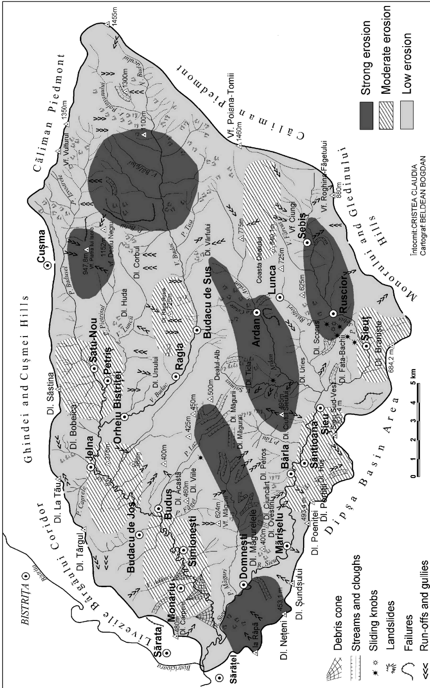
Fig. 1. Slope processes in the Șieu River Basin.
