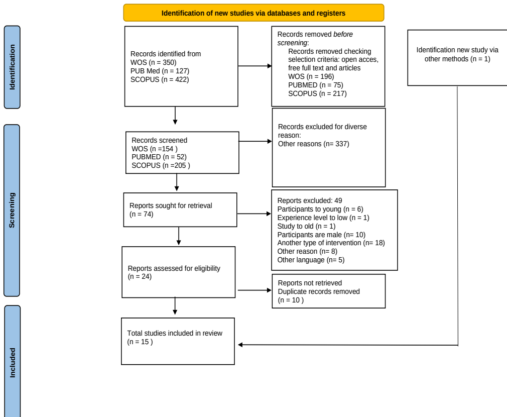
Fig. 1. Prisma Diagram
