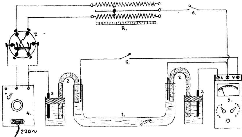
Fig. 1. Schema instalației utilizate pentru determinarea excitabilității galvanice la Idothea baltica . 1 = tubul de sticlă în U, cu \phi de 2,26 cm și lungimea eficace de 36, cm; 2 = tuburile de legătură cu paharul Berzelius cu electrolit, umplute cu agar-agar în apă de mare; 3 = electrozii de cărbune; 4 = redresor Philips legat la rețea, care furnizează un curent de 220 V.; 5 = mașetru; 6 = chei întrerupătoare; = comutator pentru inversiunea sensului curentului ce trece prin tubul U; R = rezistență reglabilă.
