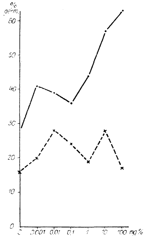
Fig. 4. Influența complexului [\text{Cr}(\text{NH}_3)_3\text{Cl}]\text{Cl}_2 asupra germinăției siclei de zahăr.
