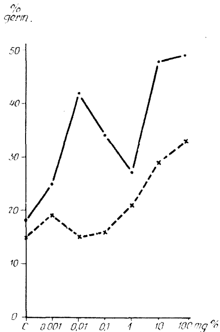
Fig. 3. Influența complexului [\text{Co}(\text{en})_3](\text{NO}_3)_3 asupra germinăției siclei de zahăr.
