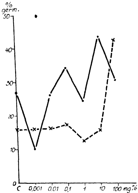
Fig. 5. Influența complexului [Cr(en)_3](SCN)_3 asupra germinatiei sfelei de zahăr.
